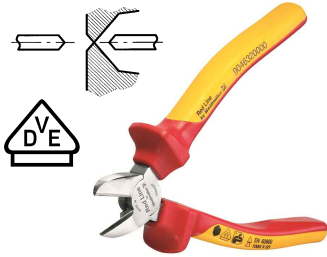
Oldalsípő fogó kemény vezetékhez
