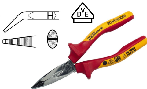
Félkerekcsőrű fogó vágóéllel (telefonfogó)
